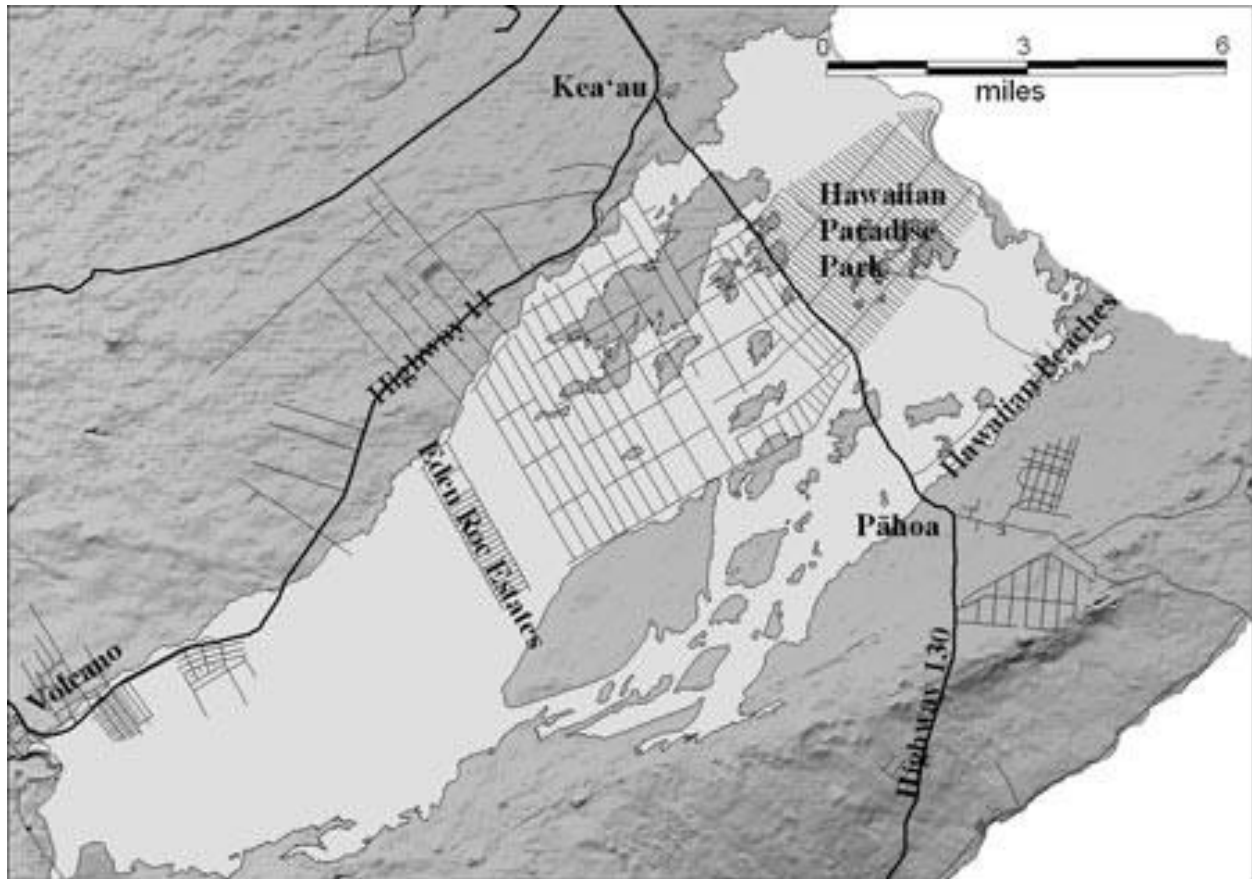
'Ailā'au Flow (light color) (USGS)
